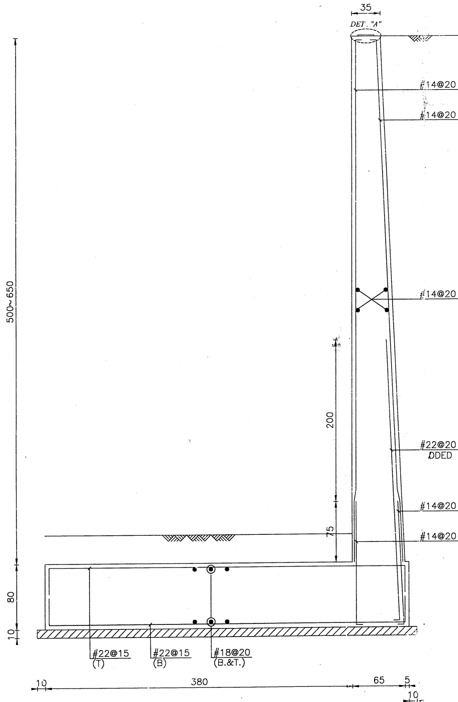
مقطع دیوار حائل با ارتفاع ۵ الی ۶٫۵ متر
