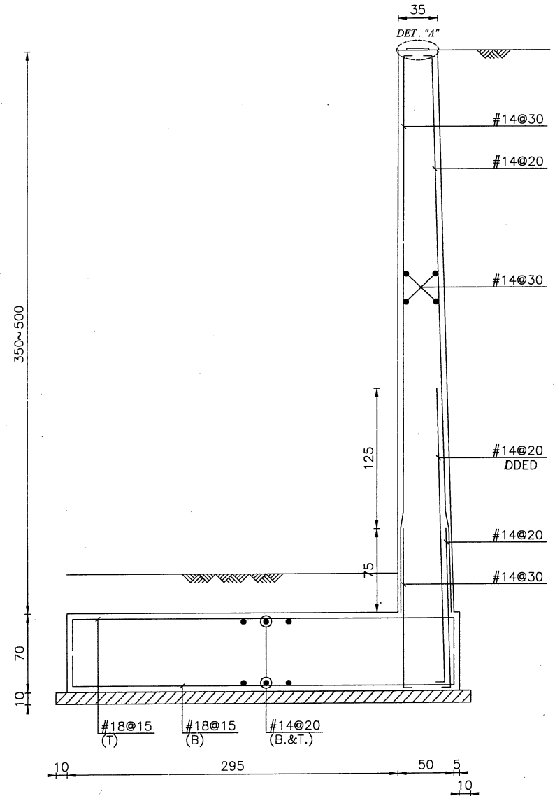
مقطع دیوار حائل با ارتفاع ۳٫۵ الی ۵ متر
